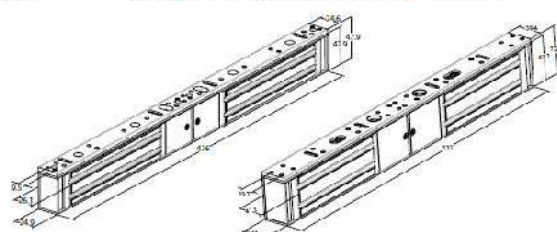
Z4 Electromagnetic Lock
