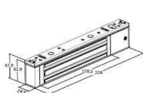
Z4 Electromagnetic Lock
